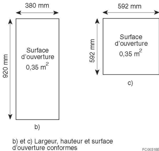
Figure A-9.7.1.3.B. Surfaces d'ouverture et dimensions des fenêtres de chambres
